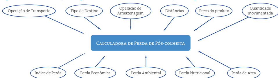
Figura 2 – Estruturação lógica da ferramenta de simulação de perdas.
